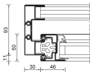
Schnitt A / Section A
